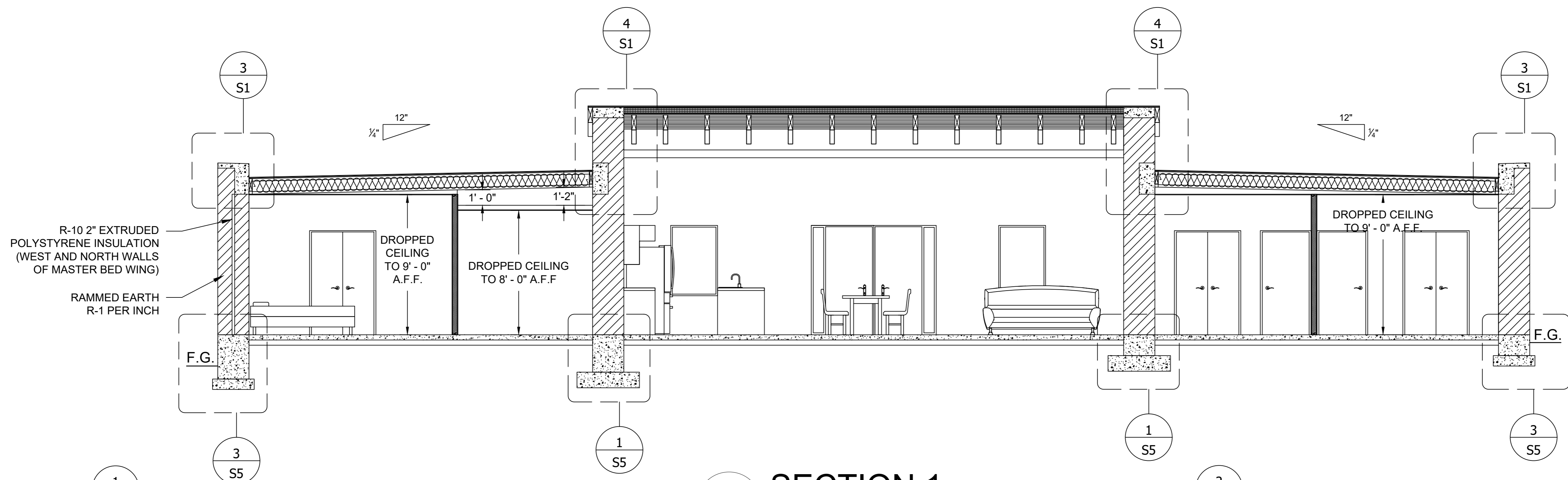
1 SECTION 1 SCALE: 1/4" = 1'-0"
