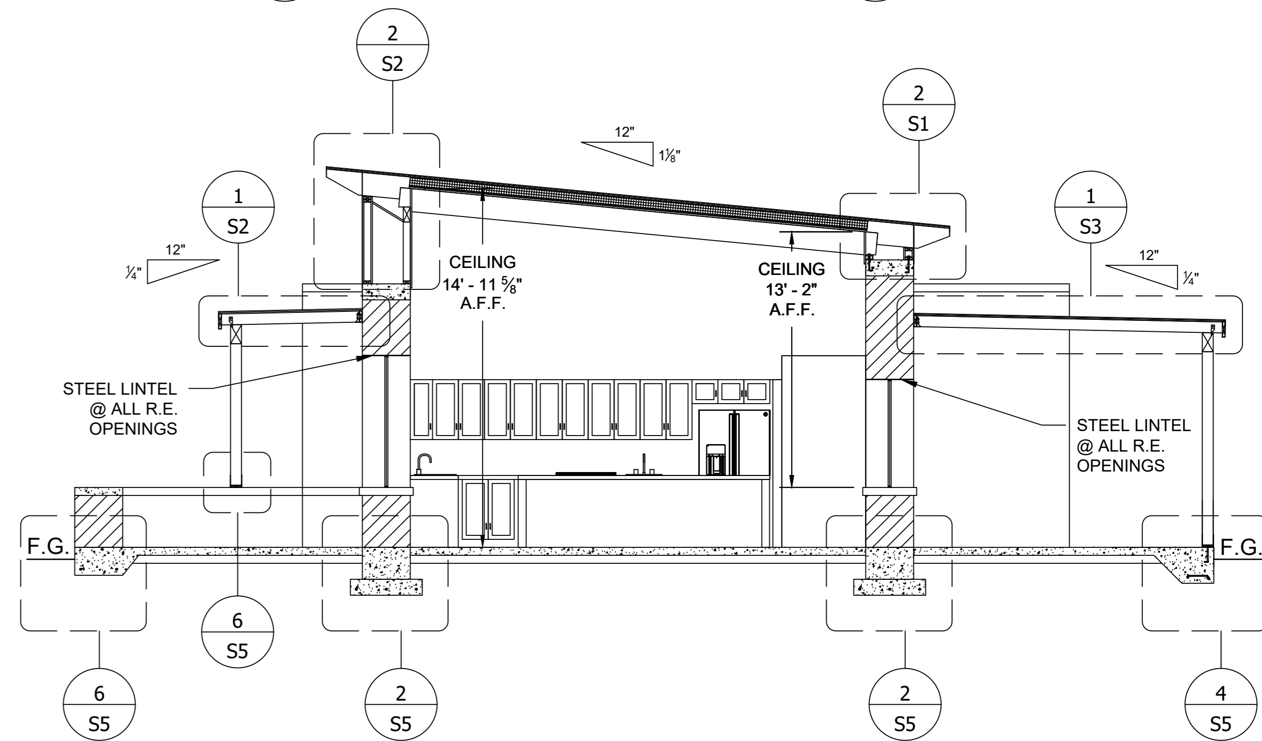
3 SECTION 3 SCALE: 1/4" = 1'-0"
