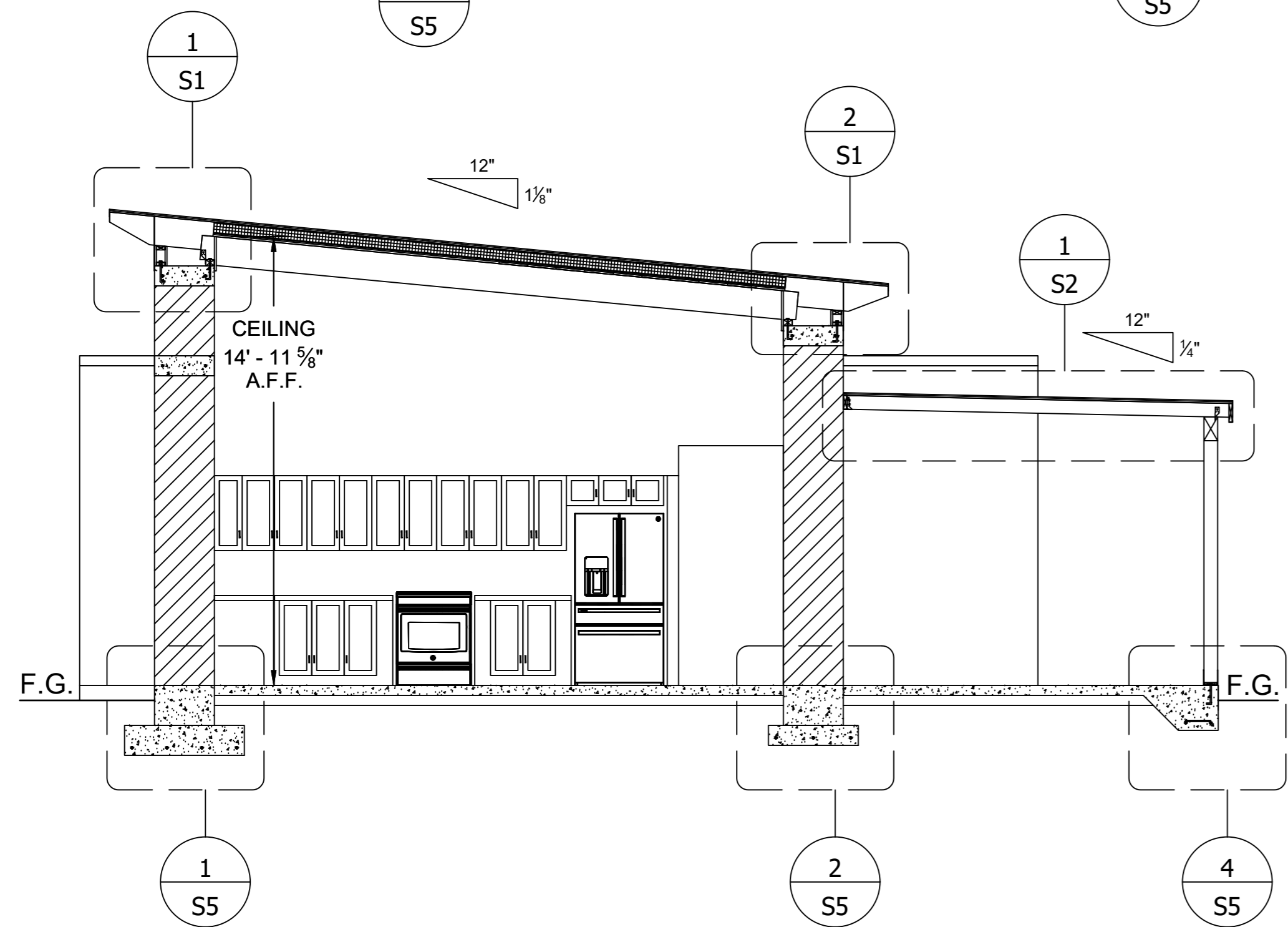
2 SECTION 2 SCALE: 1/4" = 1'-0"
